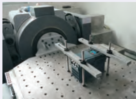
Sistema vibração elétrica
