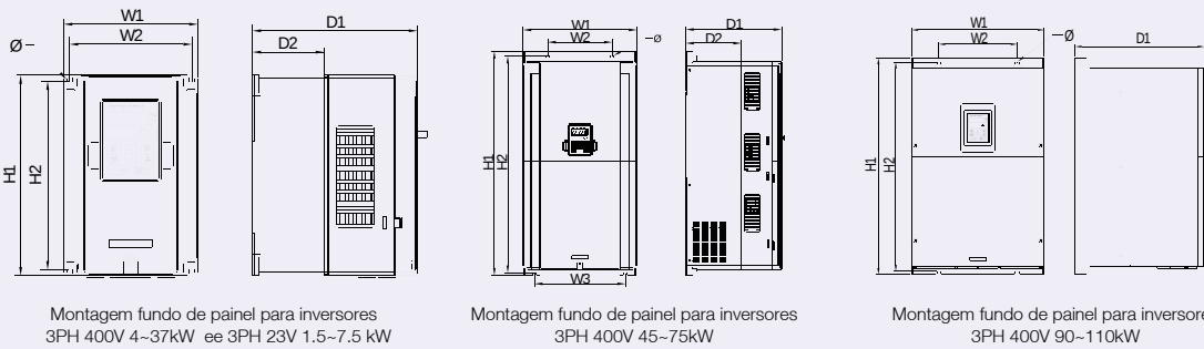
Dimensões (mm)
