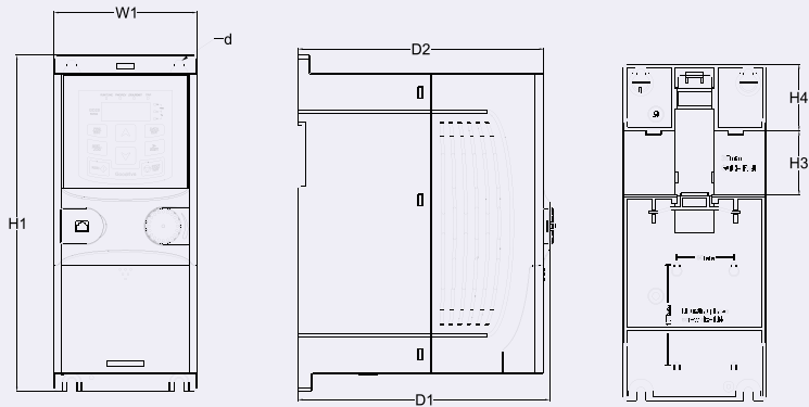
Montagem trilho DIN para inversores de 1PH 230V/3PH 400V (≤2.2kW) e 3PH 230V (≤0.75kW)
