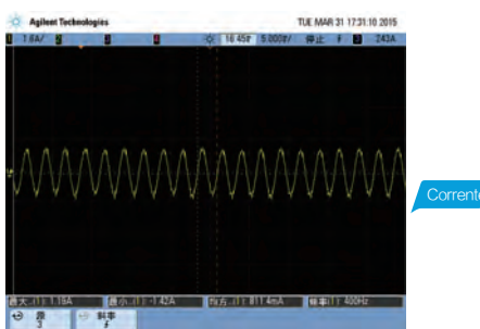
Forma de onda de corrente ao carregar subitamente no modo de controle vetorial com 0,5Hz a plena carga.
