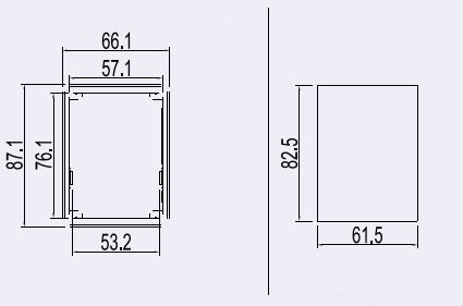
Instalação do suporte
