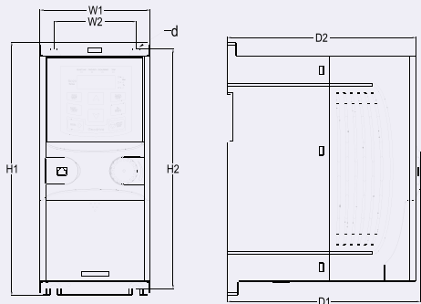
Montagem fundo de painel para inversores de 0.75~2.2kW
