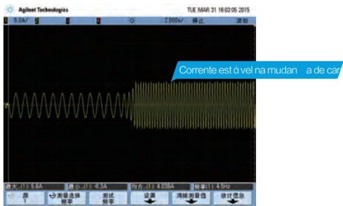
Forma de onda da corrente ao carregar subitamente no modo de controle vetorial com 0.5Hz a plena carga.
